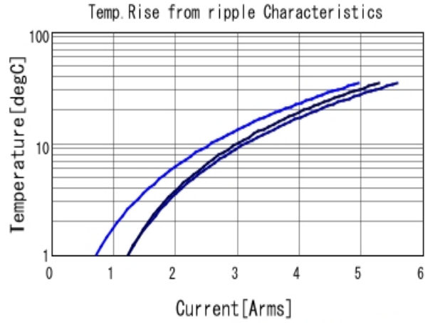
GRM188R60J226MEA0 Temp. rise ■ 80kHz ■ 400kHz ■ 800kHz
