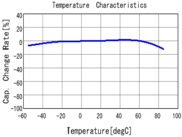
■ GRM188R60J226MEA0 C-Temp. capchange, DCO. 0V, ACO. 2Vrm
